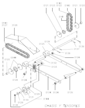
CHASIS Y TENSORES Chasis y Tensores.jpg
