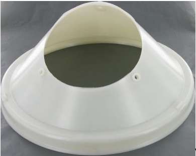
VIC0860.jpg
